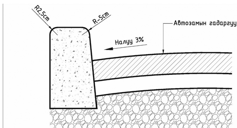
Зураг 6. Зорчих хэсгийн хийц бүтээцийн ерөнхий схем (Жишээ зураг)
