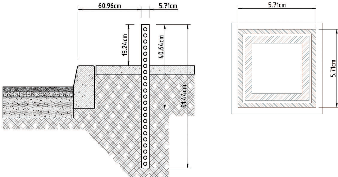
Зураг 3. Зогсоолын талбайн таних тэмдэг байрлуулах шонгийн хийц бүтээцийн ерөнхий схем (Жишээ зураг)
