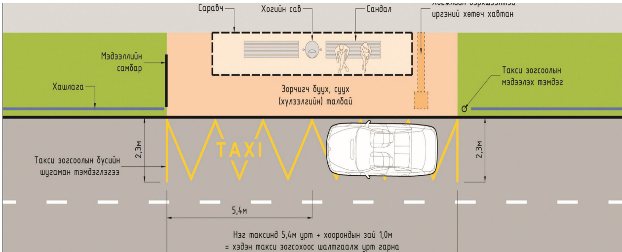
Зураг 1. Авто замын зорчих хэсэгт төлөвлөгдсөн такси зогсоолын төлөвлөлт (Жишээ зураг)
