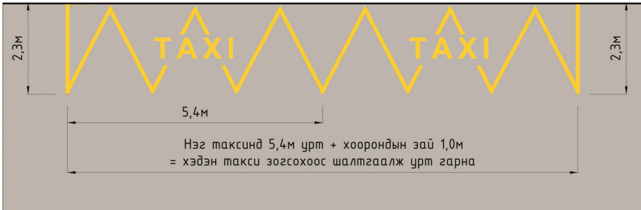
Зураг 4. Такси зогсоолын тэмдэглэгээ (Жишээ зураг)
