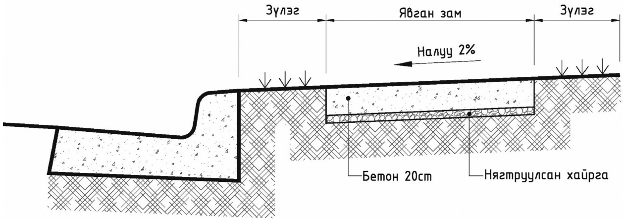
Зураг 7. Зорчих хэсэг явган замтай уялдах ерөнхий схем-1 (Жишээ зураг)
