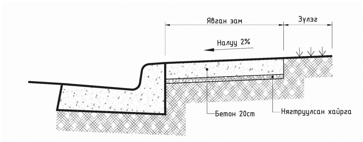
Зураг 8. Зорчих хэсэг явган замтай уялдах ерөнхий схем-2 (Жишээ зураг)
