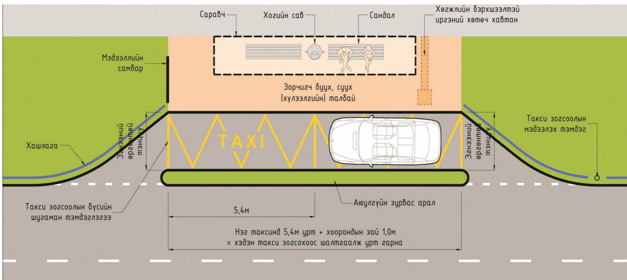
Зураг 2. Авто замын хажууд тусгаарлах зурвасаар тусгаарлагдсан такси зогсоолын төлөвлөлт (Жишээ зураг)
