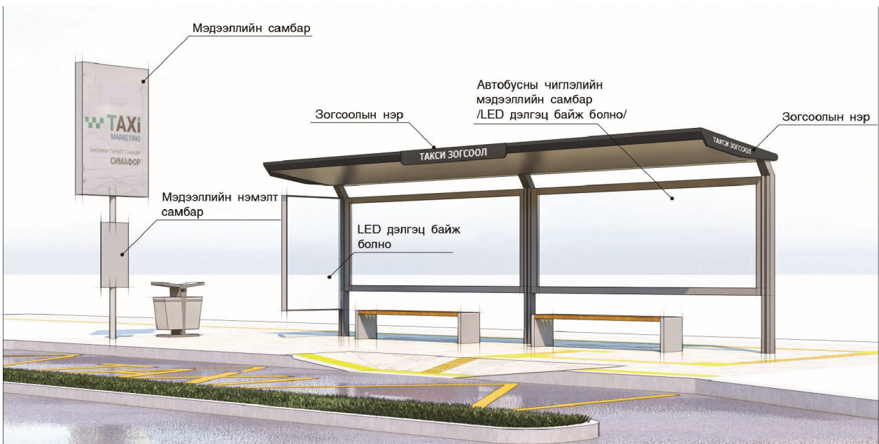
Зураг 14. Такси зогсоолын харагдах байдал (Жишээ зураг)
