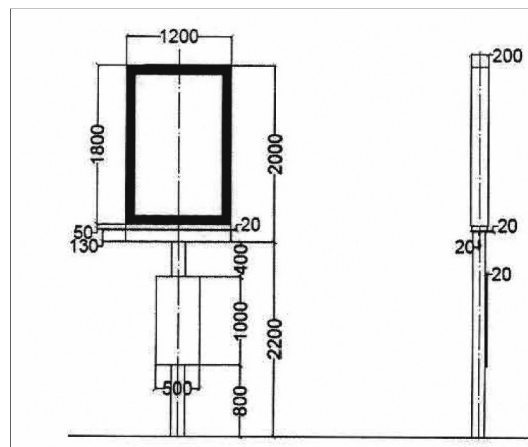
Зураг 5. Такси зогсоолын мэдээллийн самбар, хэмжээ (Жишээ зураг)
