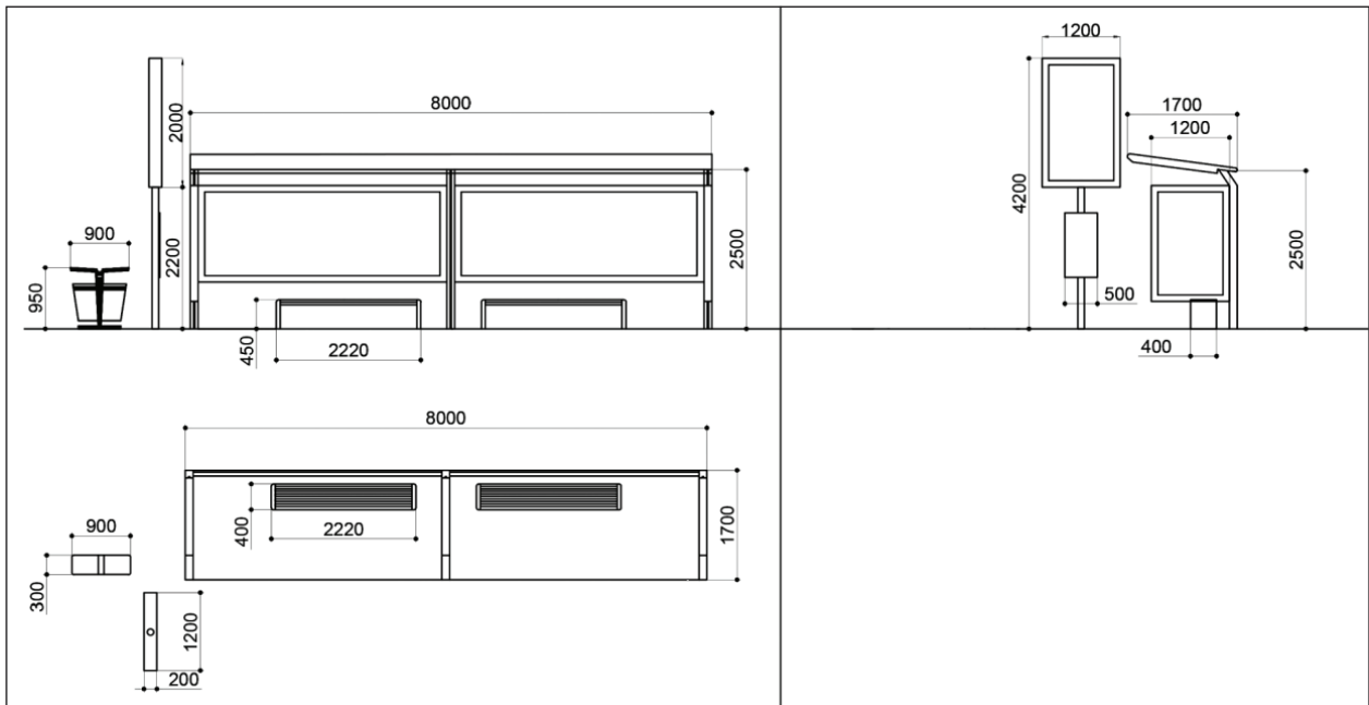
Зураг 13. Такси зогсоолын байгууламжийн хэмжээ (Жишээ зураг)
